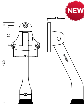
Door stop Chặn cửa móng ngựa
