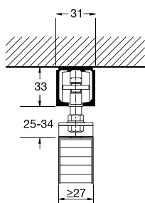
Section trolley hanger and guide Vị trí bánh xe và dẫn hướng
