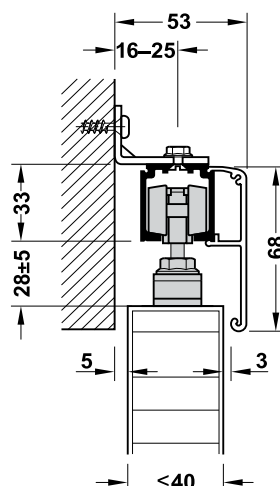
Wall mounting Gắn tường
