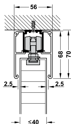
Without soft and self closing mechanism Không bao gồm giảm chấn
