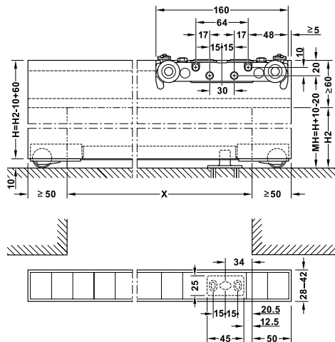
Panel preparation detail Chi tiết khoan cửa
