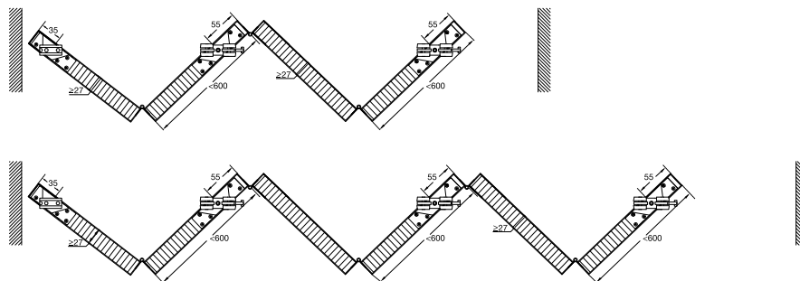
Top view installation Mặt chiếu bằng
