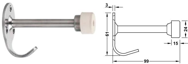
Wall mounted door stop Chặn cửa gắn tường
