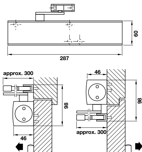
Door closer TS 4000 GEZE with standard arm Thiết bị đóng cửa tự động TS 4000 loại không giữ cửa
